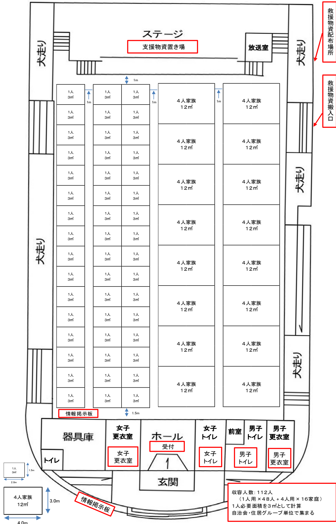
下灘小学校：体育館内配置図
