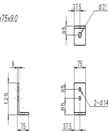
1 5 - 支柱固定金具
