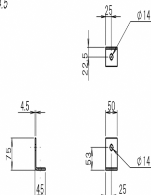
14 - 横材固定金具
