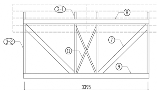
背面図
