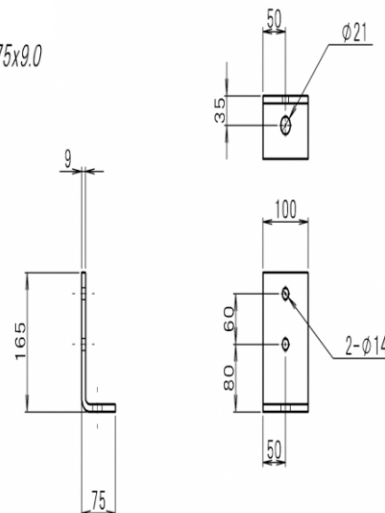
15 - 支柱固定金具
