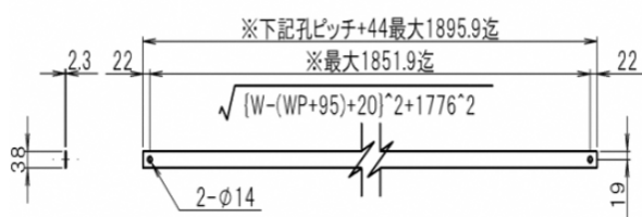
1 2 - 2 横材中央
