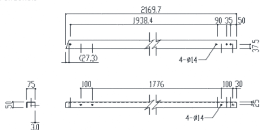
3- 1支柱後(右) 本団の勝手反対3-2支柱後(左) [-75x50x3.0]
