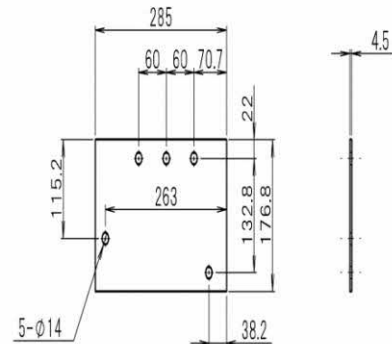
15 - 支柱固定金具
