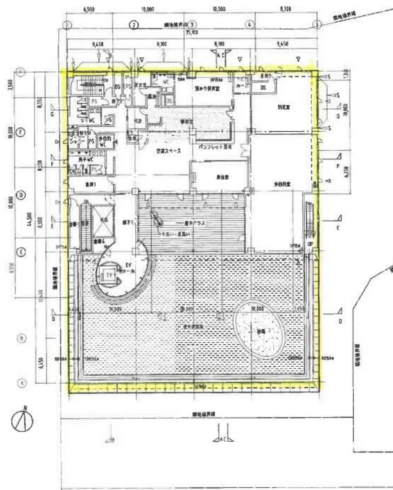
4階平面図
