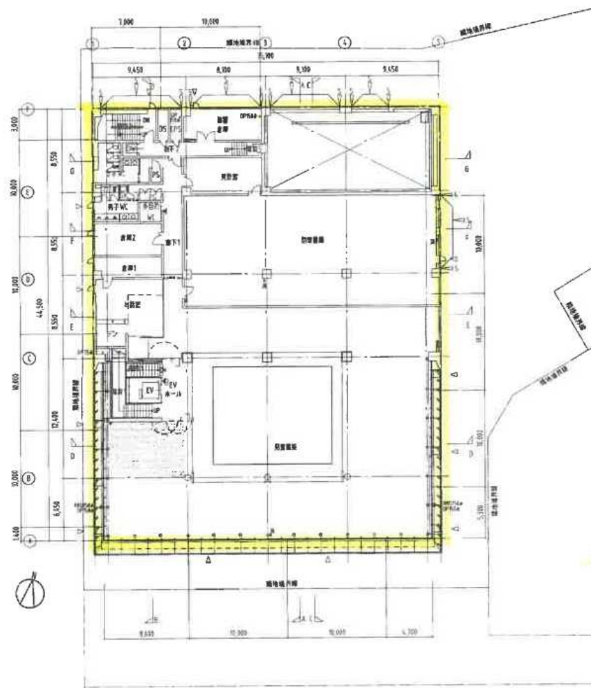
3階平面図
