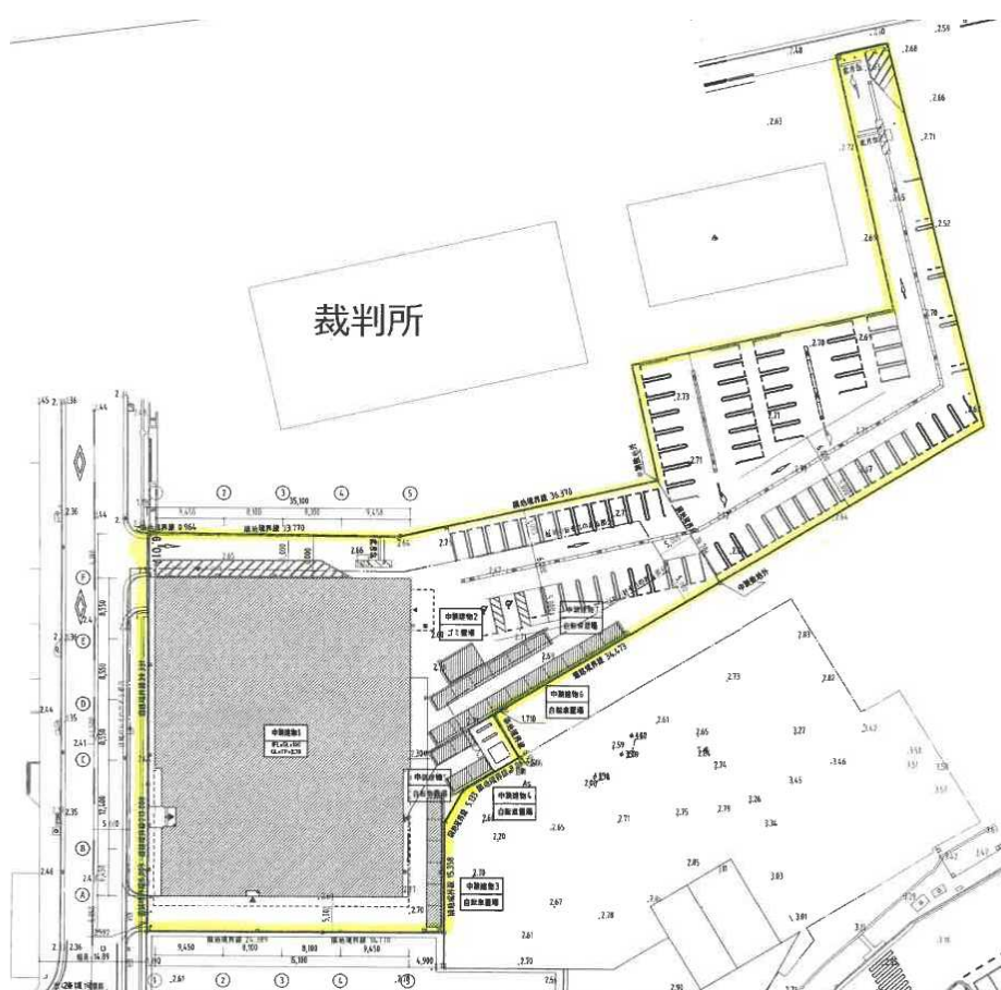
交流センター駐車場平面図
