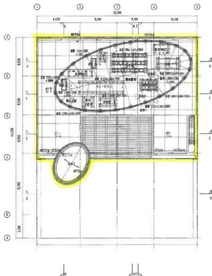
R階平面図
