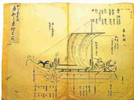
車舟の図(蒸気船を作る途中で参考にした実験用の船の絵図) (公財)宇和島伊達文化保存会
