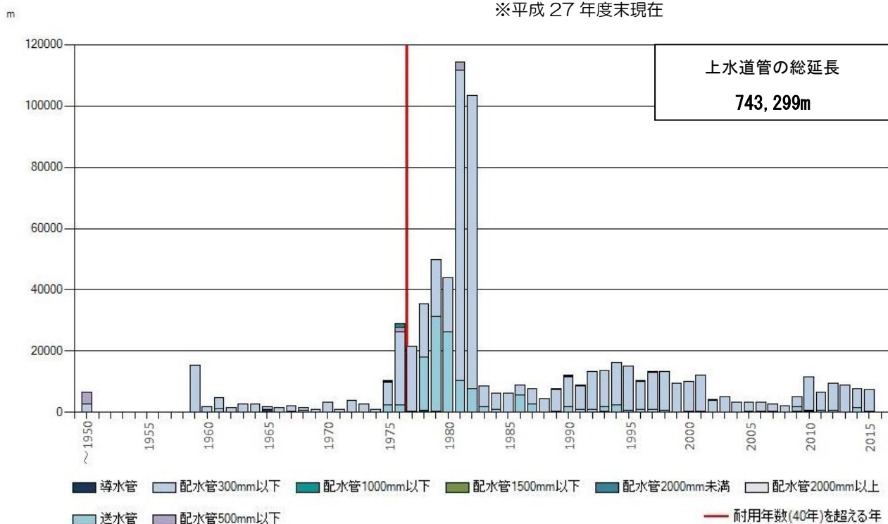
図 2.12 上水道管の管種別整備年度別延長
