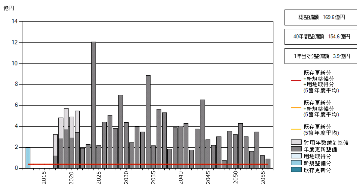
図6.2 橋りょうの更新等費用の推計
