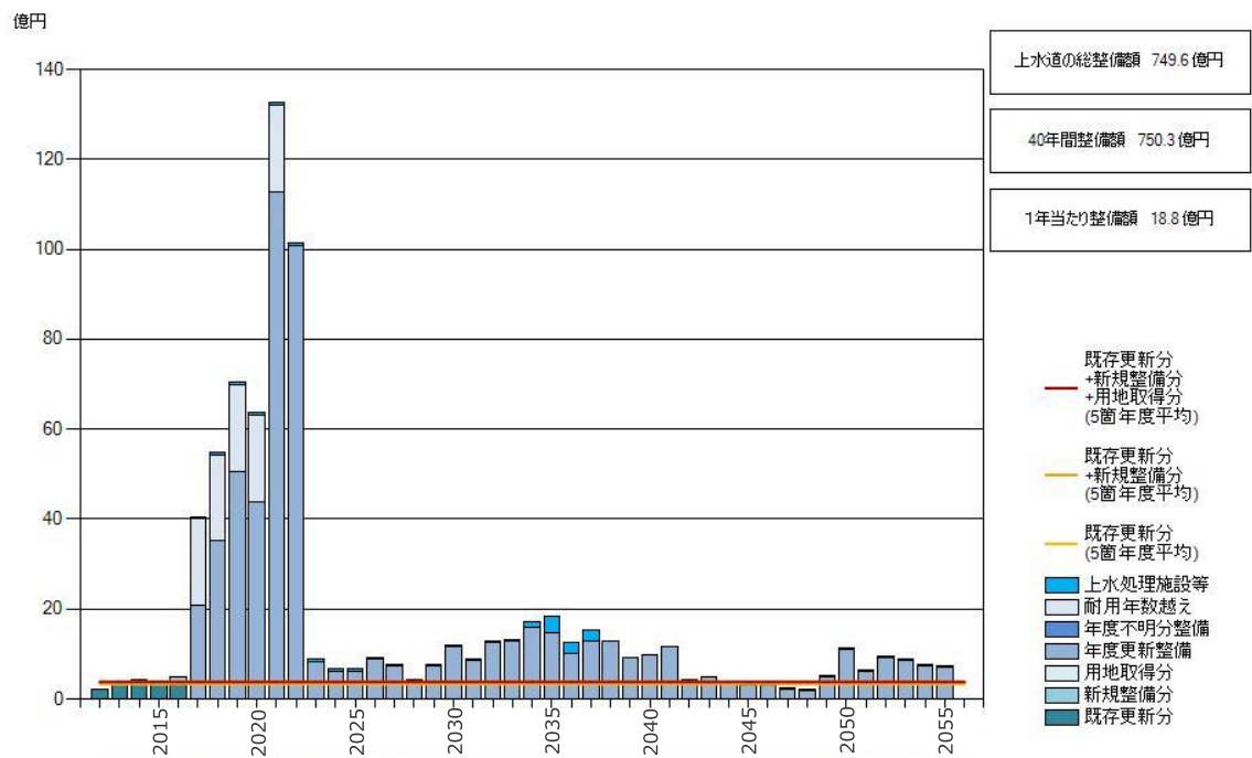
図6.3 上水道施設の更新等費用の推計
