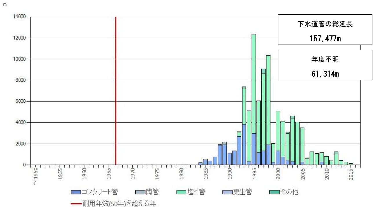
図 2.13 下水道管の管種別整備年度別延長
