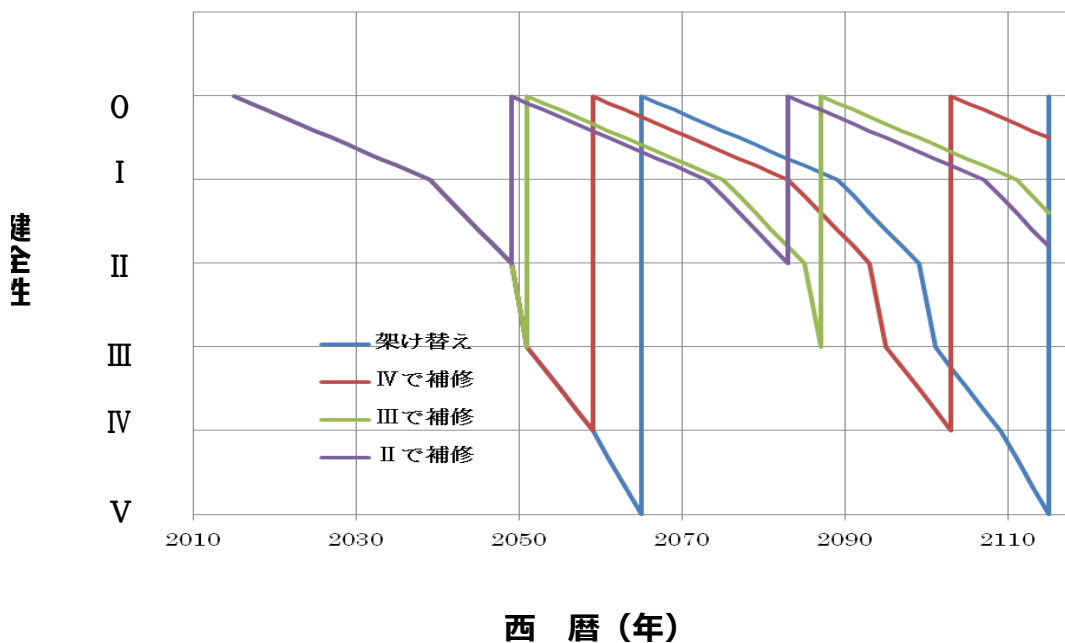
図-2 健全性の低下の例（劣化曲線）
